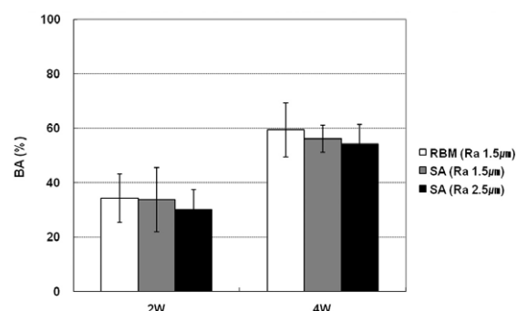
Fig. 3. BA analysis.
